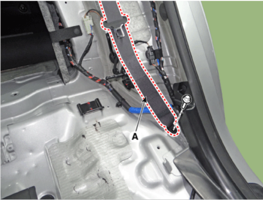
8. 拆卸后安全带弯曲盖(A)。
